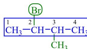
2-bróm-3-metilbután
