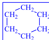
ciklohexán
