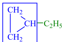
etilciklopropán
