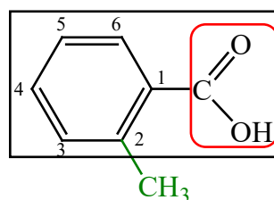
2-metilbenzoészav
