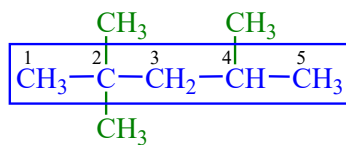
2,2,4-trimetilpentán
