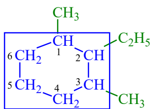
2-etil-1,3-dimetilciklohexán
