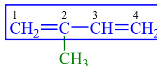
2-metilbuta-1,3-dién
