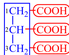
propán-1,2,3-trikarbonsav
