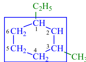
1-etil-3-metilciklohexán
