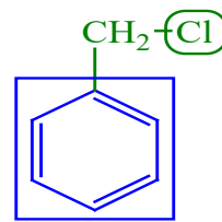
(klórmetil)benzol
