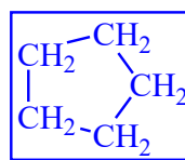
ciklopentán
